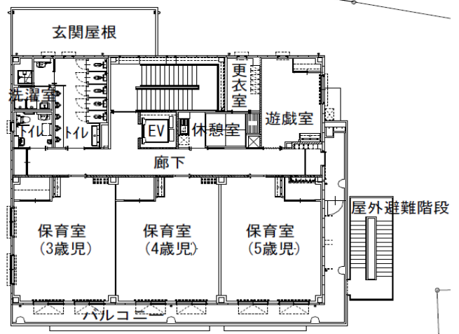
2F平面図
