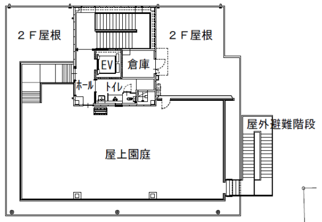
3F平面図
