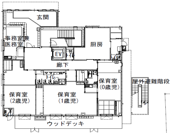
1F平面図
