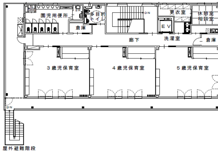
2階平面図
