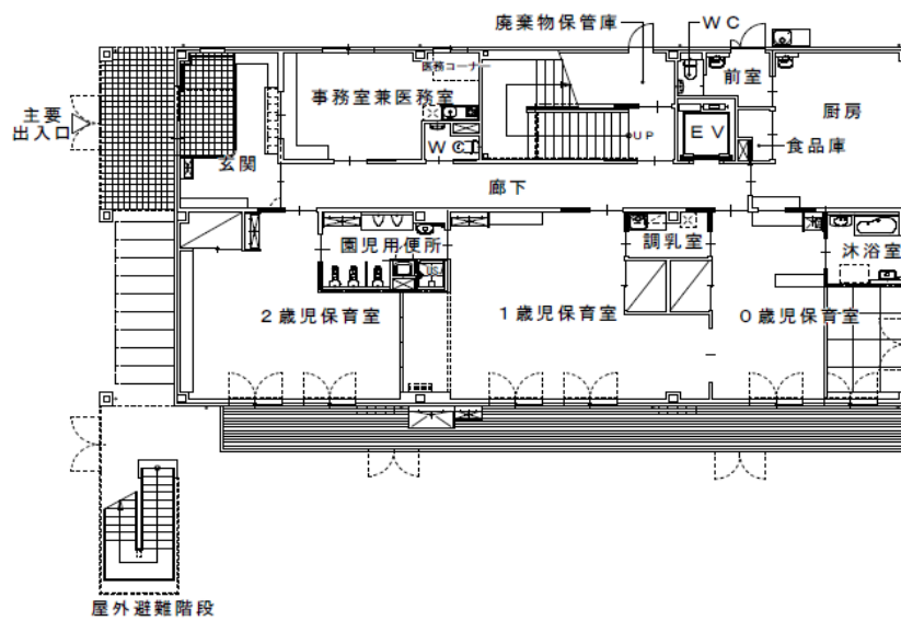
1階平面図
