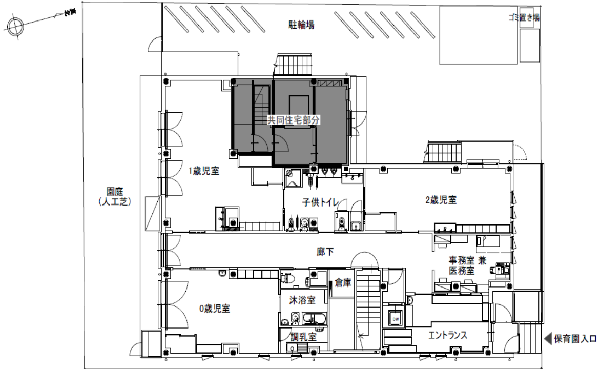
【1階平面図】
