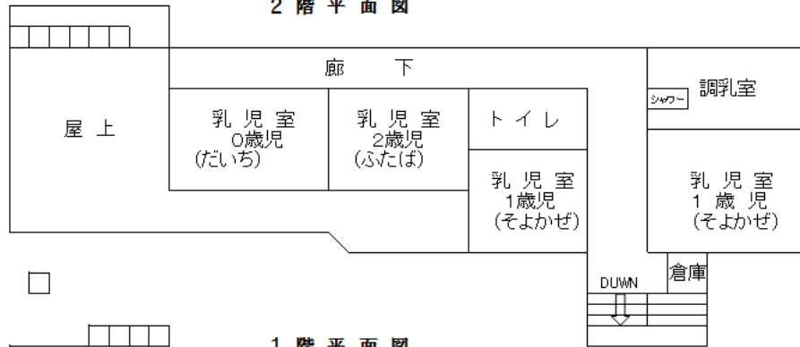
1階平面図
