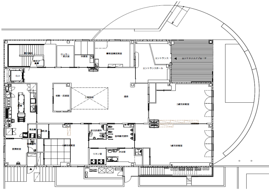
1F平面図
