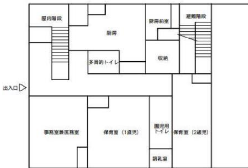
1階
